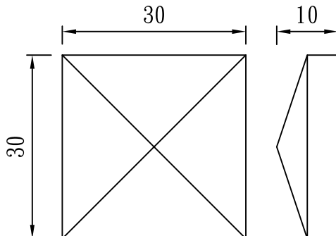
型號：DF-W30T3H30
