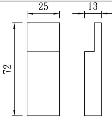
型號：DF-257213
