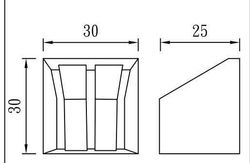
型號：DF-303005
