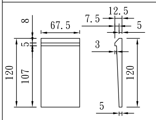
型號：DF-6813120
