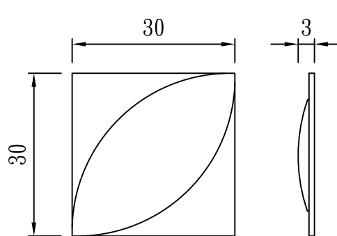
型號：DF-W30T3H30
