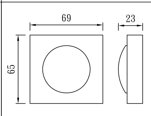
型號：DF-696523
