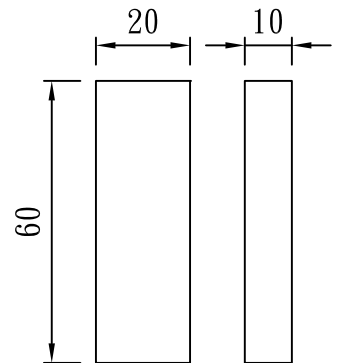
型號：DF-206010
