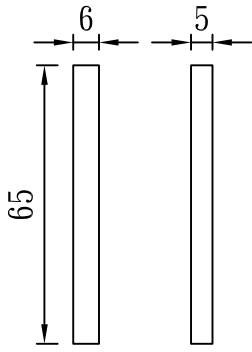
型號：DF-W6T5H65
