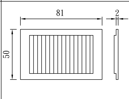
型號：DF-815004
