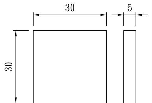
型號：DF-303005
