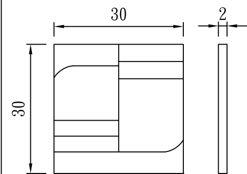
型號：DF-W30T2H30
