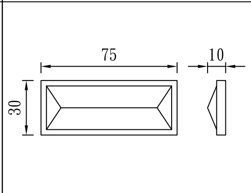
型號：DF-W75T10H30
