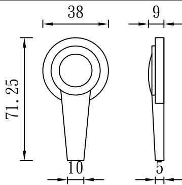
型號：DF-257213
