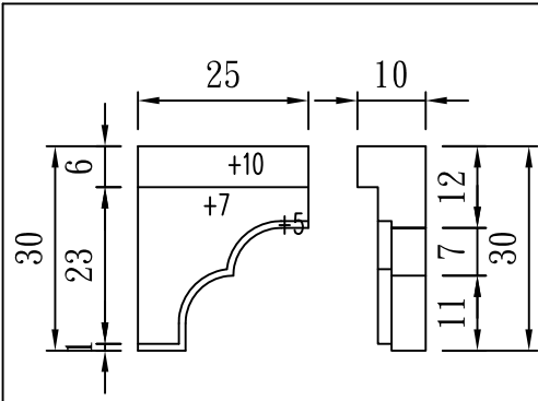
型號：DF-W25T10H30
